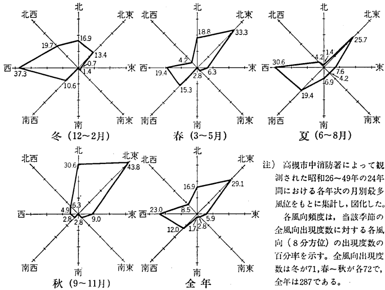
図43 高槻の風向
