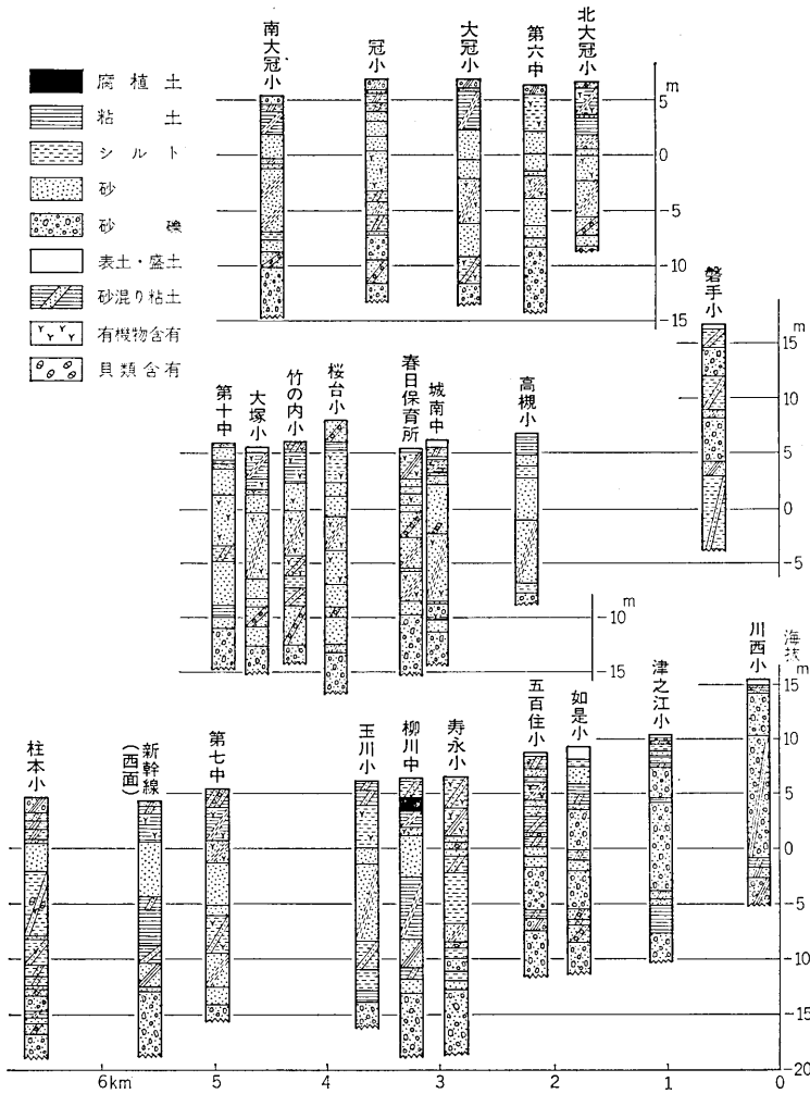
図22 淀川低地の地質柱状図
