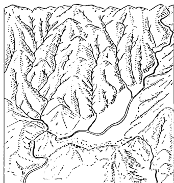
C 現在の状態
