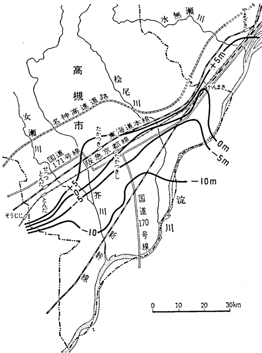
図38 淀川低地における沖積層基底等深線図
