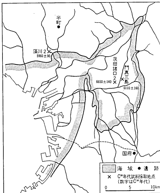
図34 河内湾Ⅰの時代(約7,000～6,000年前、縄文時代前期前半)の古地理図 (梶山彦太郎・市原実・前掲論文による)
