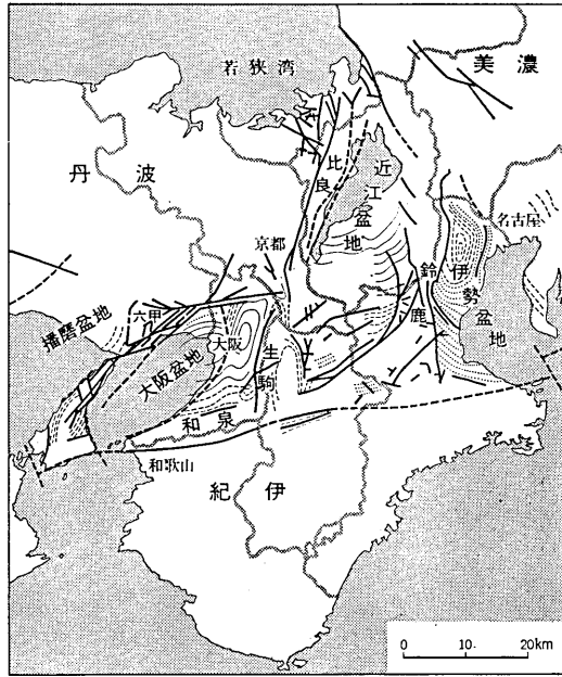
図30 近畿三角地帯の地質構造 (IKEBE & ICHIKAWA) 太線は六甲変動にともなう断層系を、細線は大阪層群相当層 (大阪層群, 古琵琶湖層群, 東海層群など) のだいたいの走向方向を示す (点線: 最下部, 破線: 下部, 実線: 上部)
