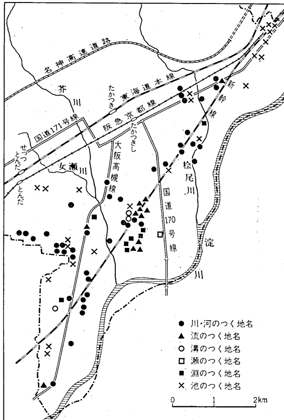
図40 淀川低地における河川・湿地関係地名の分布
