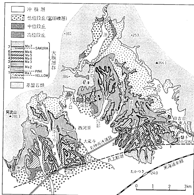
図19 高槻北方丘陵の地質 (西山団体研究グループ・桂高校地学クラブ「高槻地方丘陵 の大阪層群」『地球科学』24—6, 1970年による)
