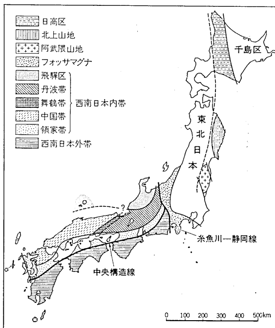
図23 日本列島の地体構造区分 (中野尊正・小林国夫『日本の自然』岩波新書を簡略化)
