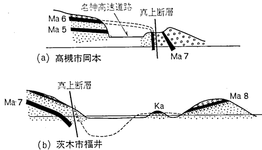
図20 真上断層の模式断面 (西山団体研究グループ他・前掲論文による)
