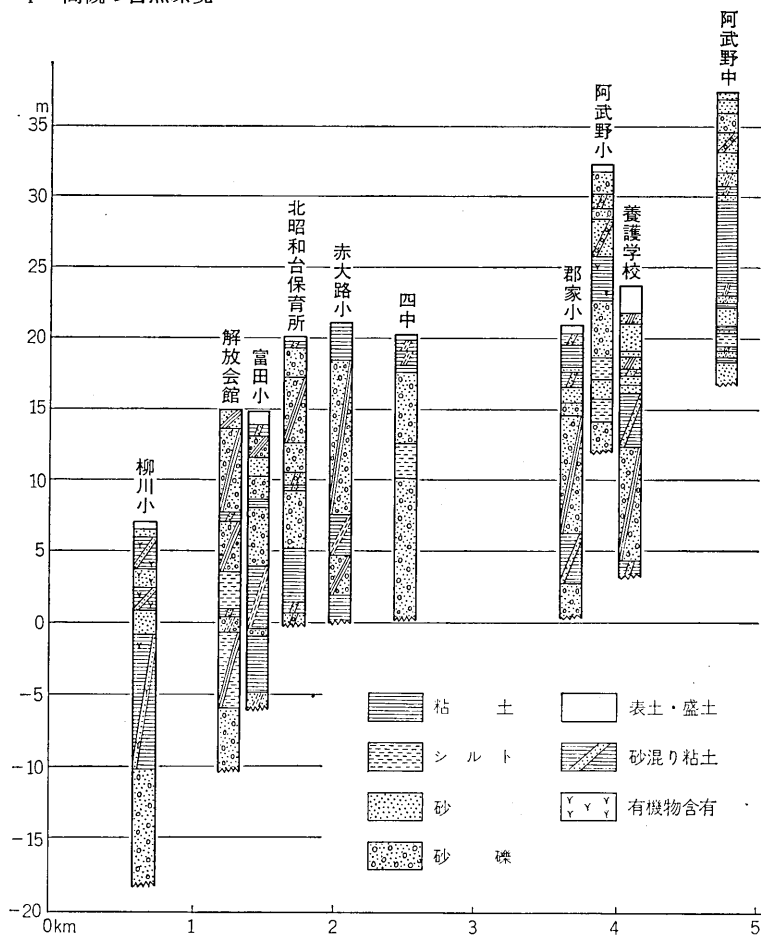
図31 富田台地の地質柱状図
