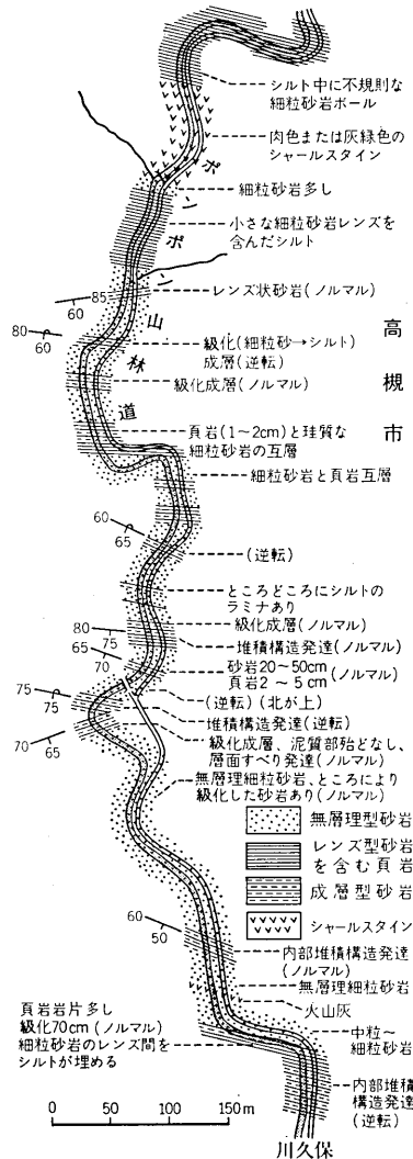
図17 水無瀬川河谷の地質図
