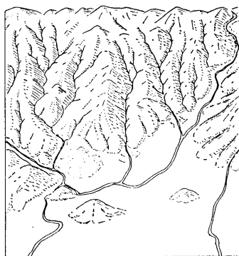
B 侵食が開始された時の状態
