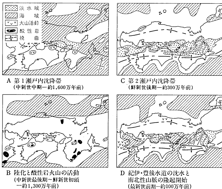
図27 瀬戸内沈降帯形成期の古地理図 (市原実「大阪層群と六甲変動」(前掲)による)
