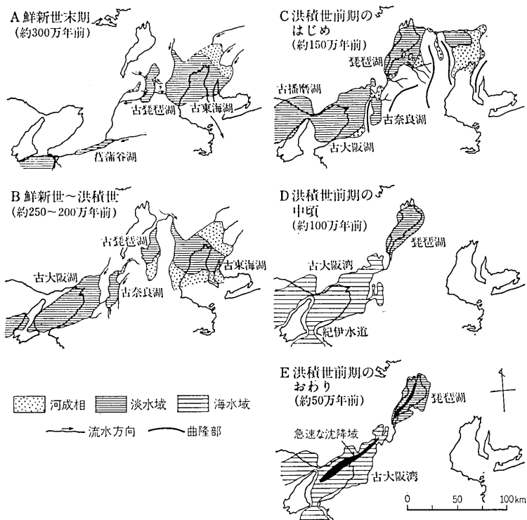
図28 大阪層群堆積期の古地理の変遷
