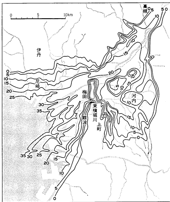
図33 大阪平野の沖積層基底等深線図 （梶山彦太郎・市原実「大阪平野の発達史」『地質学論集』第7号、1972、による）
