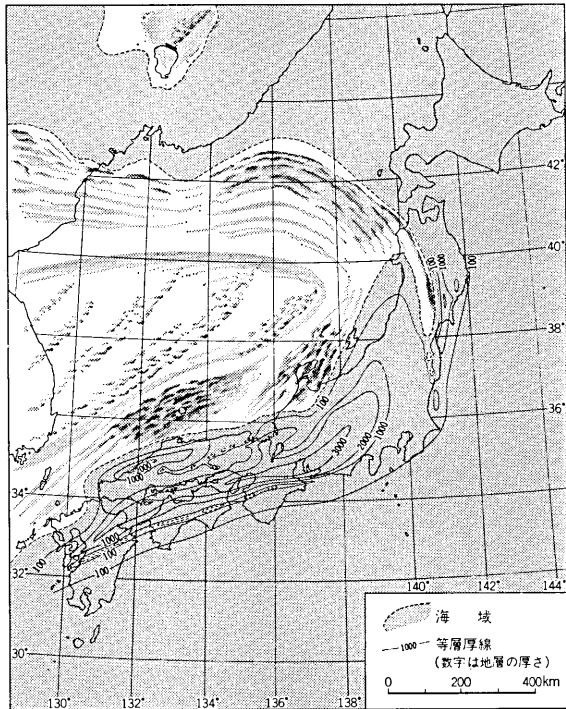
図25 ペルム紀後期(約2億4,000万年前)の古地理図 (市川浩一郎・藤田至則・島津光夫編『日本列島地質構造発達史』, 築地書館, 昭和45年による)
