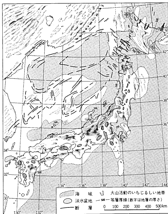
図26 中新世末期(約1,400万年前)の古地理図 (市川浩一郎他, 前掲書, による)
