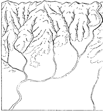
A 大阪層群堆積当時の状態
