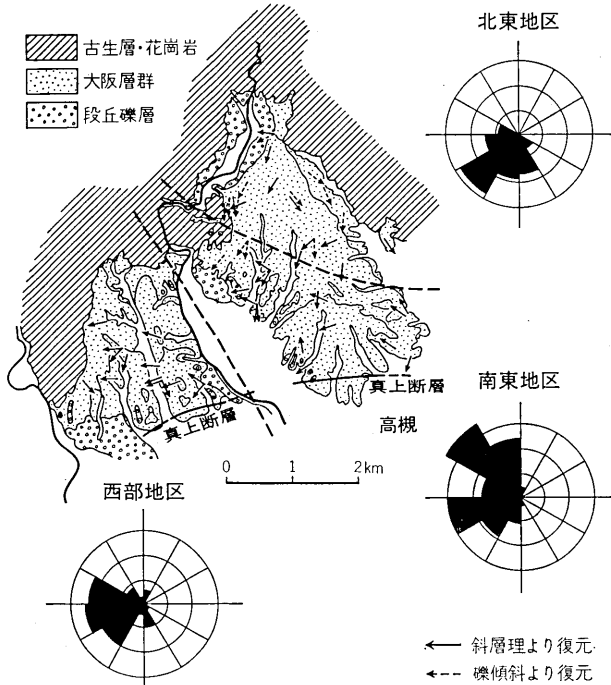
図29 高槻丘陵における大阪層群堆積当時の古水流方向 (YOKOYAMA, T. 前掲論文による)
