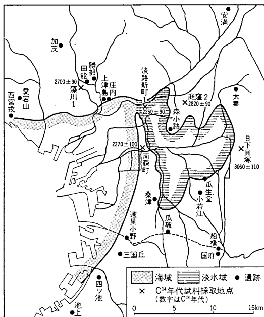
図36 河内潟の時代(約3,000～2,000年前, 縄文時代後期～弥生時代前期)の古地理図 (梶山彦太郎・市原実, 前掲論文による, 一部修正)
