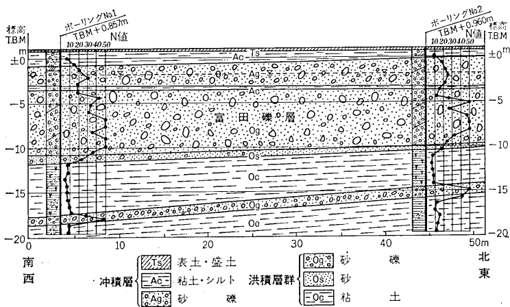
図21 富田礫層の地質断面 (応用地質調査事務所『富田小学校体育館 増築工事に伴う土質調査』1968年による)
